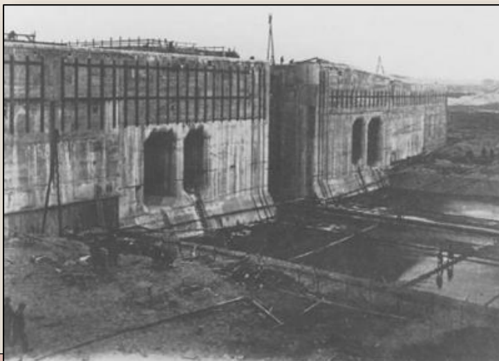
De bouw van de nieuwe schutsluis te IJmuiden (circa 1924)
