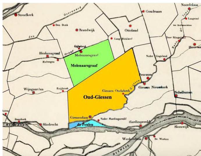
Afb. 1. Alblasserwaard met de relevante ambachtsheerlijheden.
